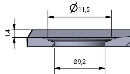
Detalle B
