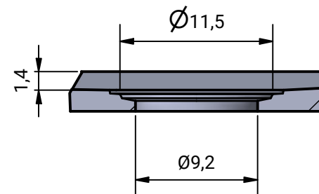
Detalle B
