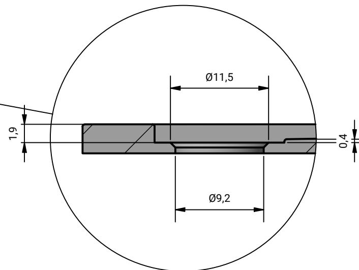
Detalle E
