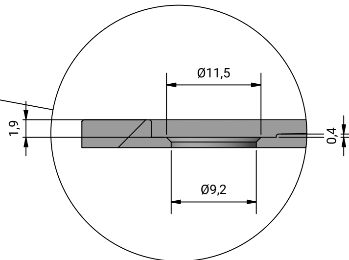
Detalle E
