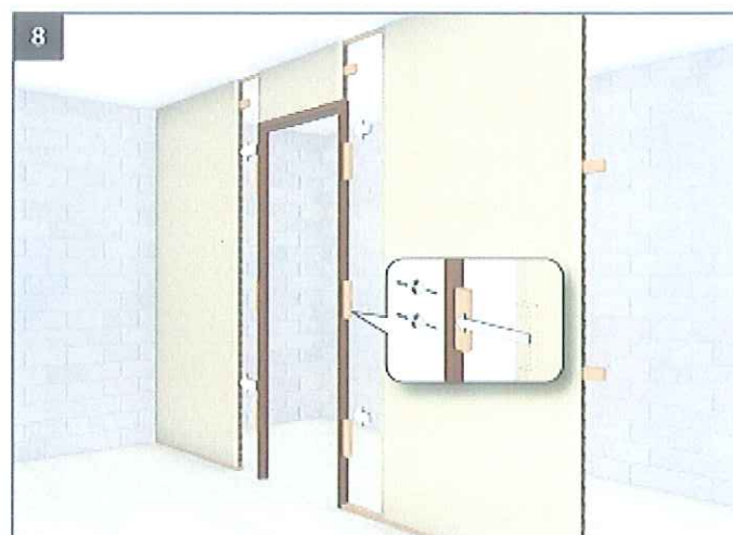
Figure 8 – Mise en œuvre de d'une huisserie
