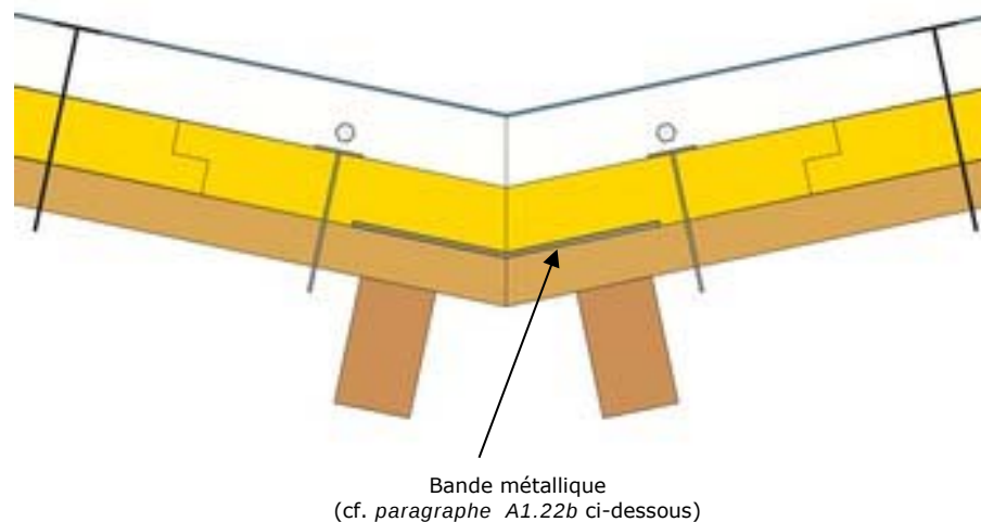
Figure 10 – Principe de jointoiement du procédé Stisolétanc® Protect avec élément porteur bois - panneaux à base de bois, sur appui double de la noue en bois
