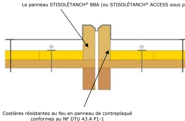
Figure 29 – Exemple du traitement au droit d'un joint de dilatation sur élément porteur bois - panneaux à base de bois, avec des costières résistantes au feu en panneau de contreplaqué
