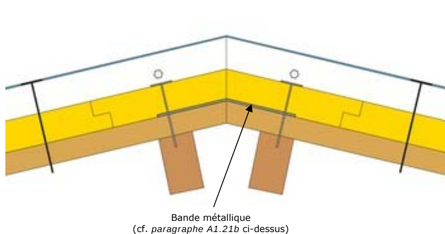
Figure 9 – Principe de jointoiement du procédé Stisolétanc® Protect avec élément porteur bois - panneaux à base de bois, sur appui unique du faîtage ou arêtier
