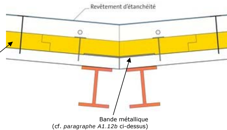
Figure 8 – Principe de jointoiement du procédé Stisolétanc® Protect avec élément porteur tôle d'acier nervurée, sur appui double de noue traditionnelle
