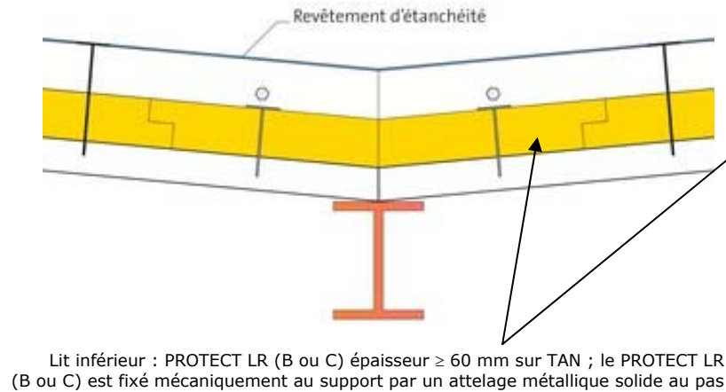
Figure 7 – Principe de jointoiement du procédé Stisolétanch® Protect avec élément porteur tôle d'acier nervurée, sur appui unique de noue traditionnelle
